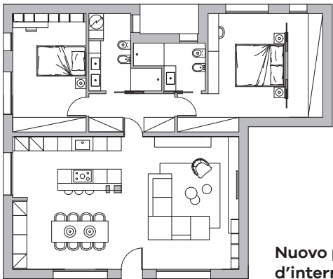
Modifiche disposizione interna pareti
